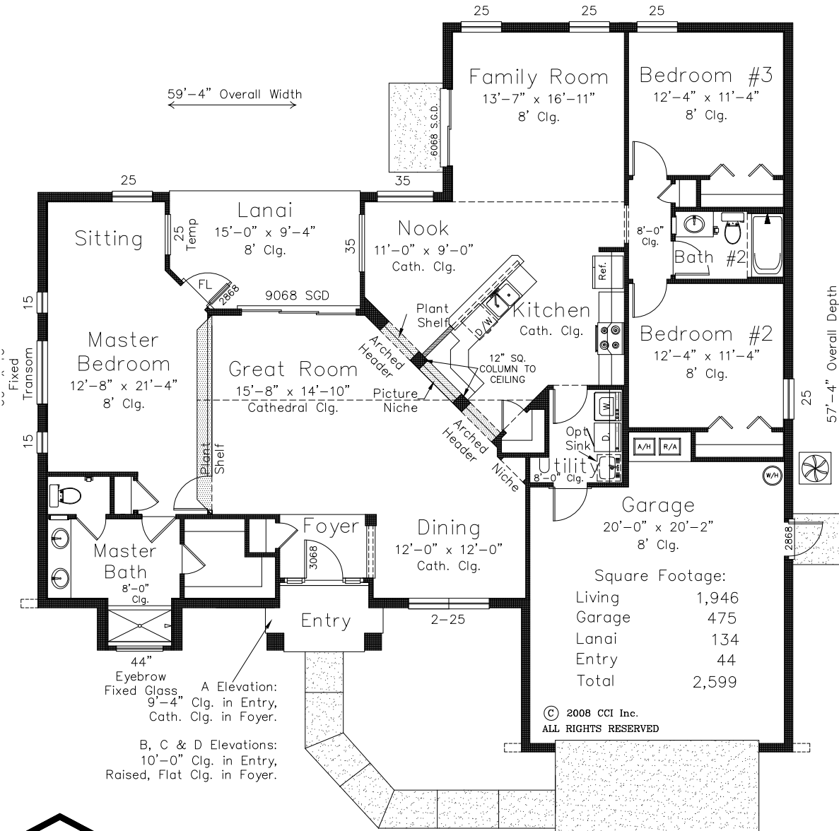
Elevation "C"
