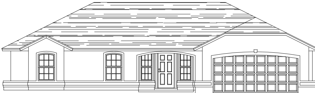
Elevation "C"
