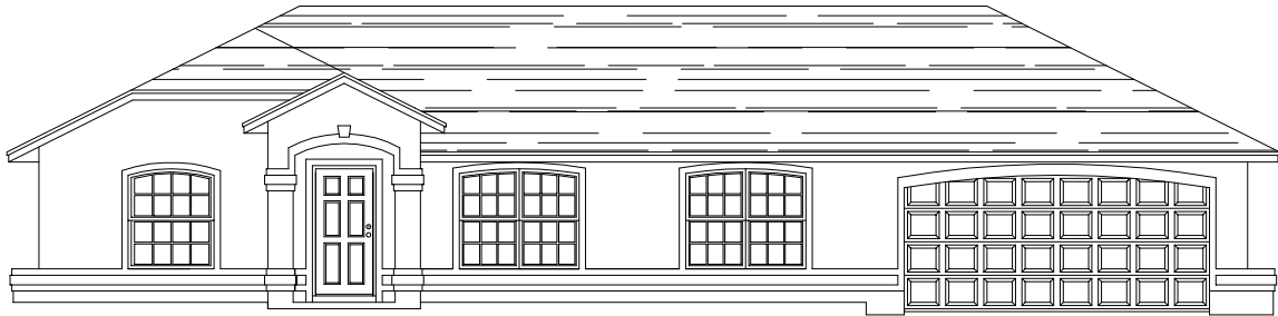
Elevation "C"
